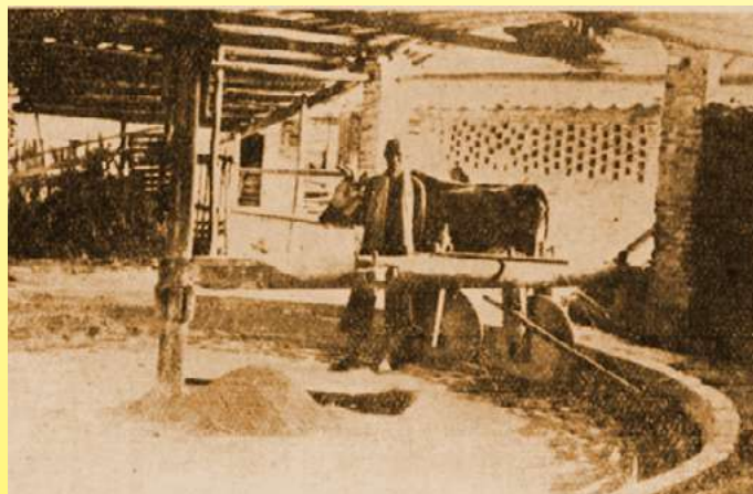
Macinazione del caolino con macine azionate da un bue (1939, Vietnam, Economic Bulletin of Indo-China)
