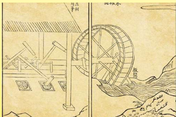
Ruota ad acqua e martello da viaggio (水碓 shui duì) per la macinazione dei minerali (Tiangong Kaiwu, Song Yingxing 1637)
