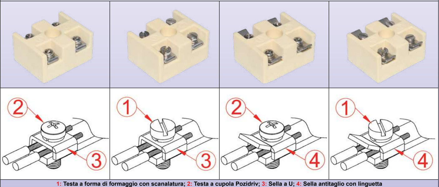
1: Testa a forma di formaggio con scanalatura; 2: Testa a cupola Pozidriv; 3: Sella a U; 4: Sella antitaglio con linguetta
