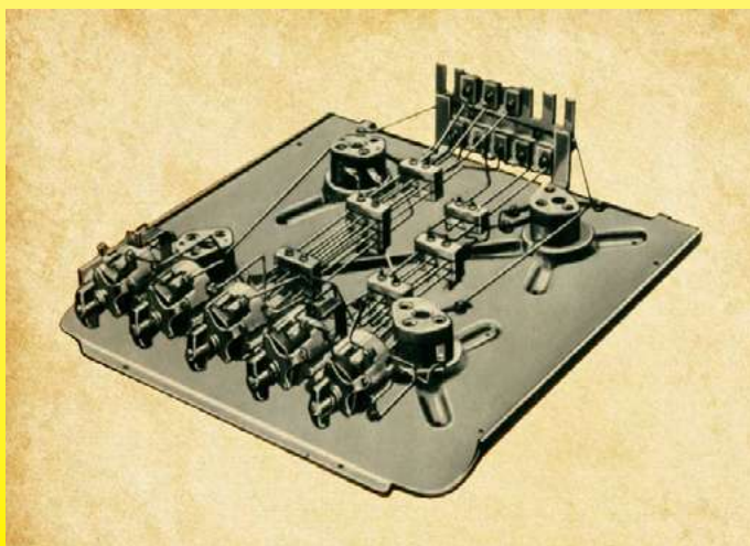
Cablaggio elettrico del piano di una stufa elettrica Arthur Martin (Catalogo 1949, Ultimheat Museum). I pezzi isolanti in steatite e porcellana sono onnipresenti
