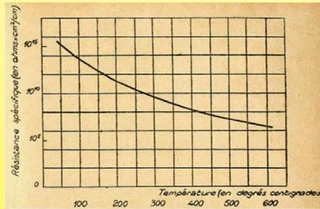
Variation della resistenza specifica in ohm.cm/cm 2 della porcellana in funzione della temperatura (curva logaritmica). Tra 20°C e 300°C la sua resistenza è divisa per 10,000 (1945 Matériaux électrotechniques modernes, Ultiheat Museum).
